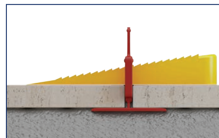
Clip plat LASH® pour les carreaux de sol et mur
